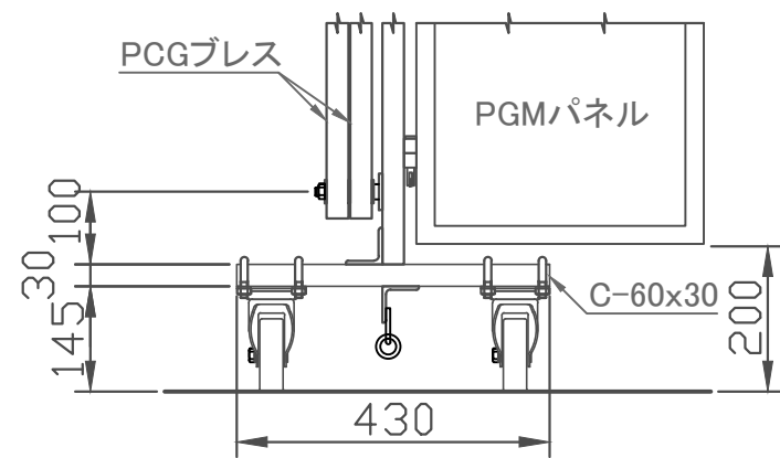
走行棒下部詳細
