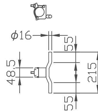
丁番クランプ詳細
