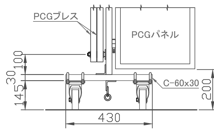
走行棒下部詳細
