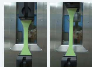
JIS A 6021引張性能試験の例
