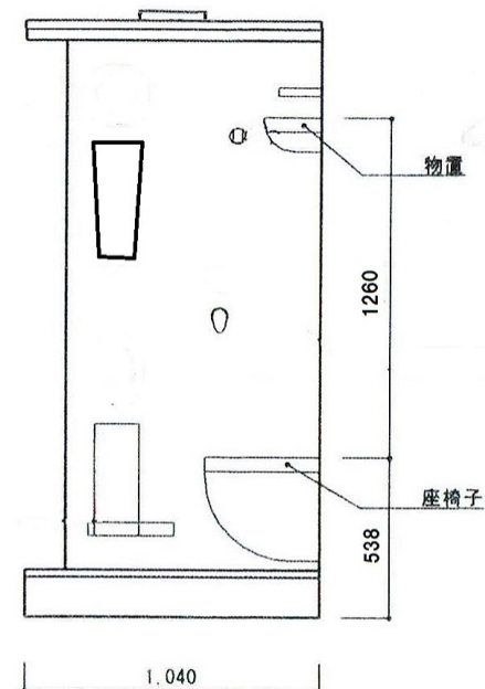
側面内部
