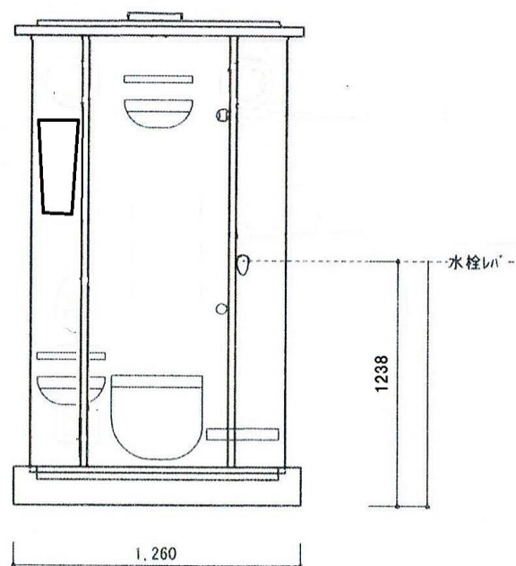
正面内部
