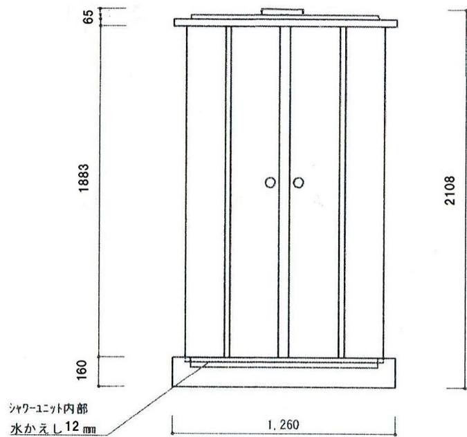
正面外観
