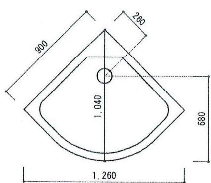
床平面図
