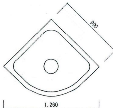
天井平面図(内側)
