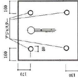
床底面図 S=1/20
