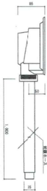
排水トラップ S=1/5
