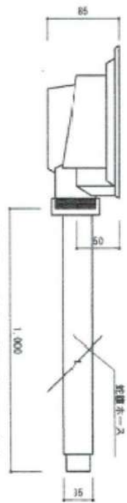
排水トラップ S=1/5
