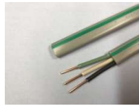
600Vビニル絶縁ビニルシー スケール平形 黒・白・緑 2mm-3心
