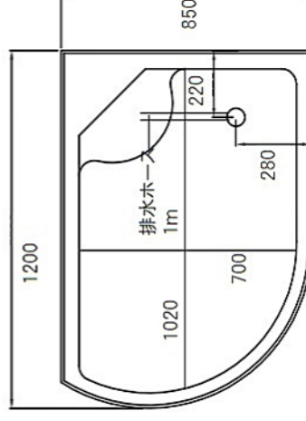
床パネル ↓正面側 (上部より) 浴槽深さ350
